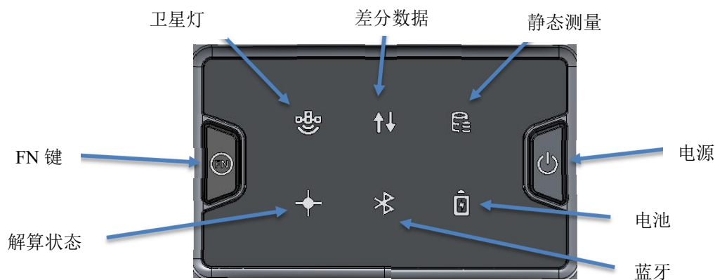
图 1.4 基础版的按键和 LED 灯
