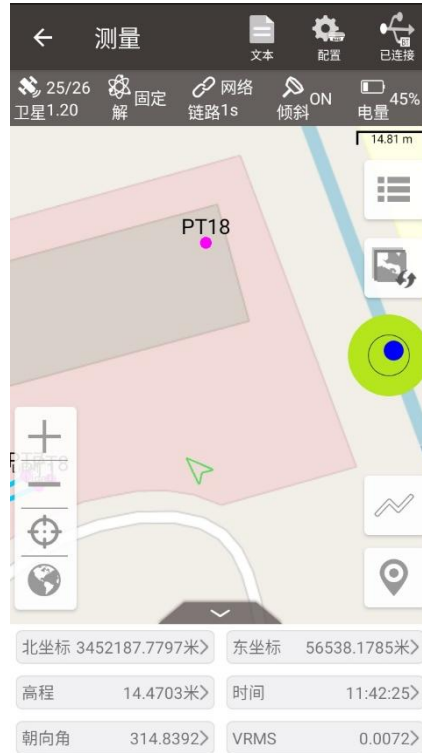
图 4.24 倾斜补偿状态已开启
