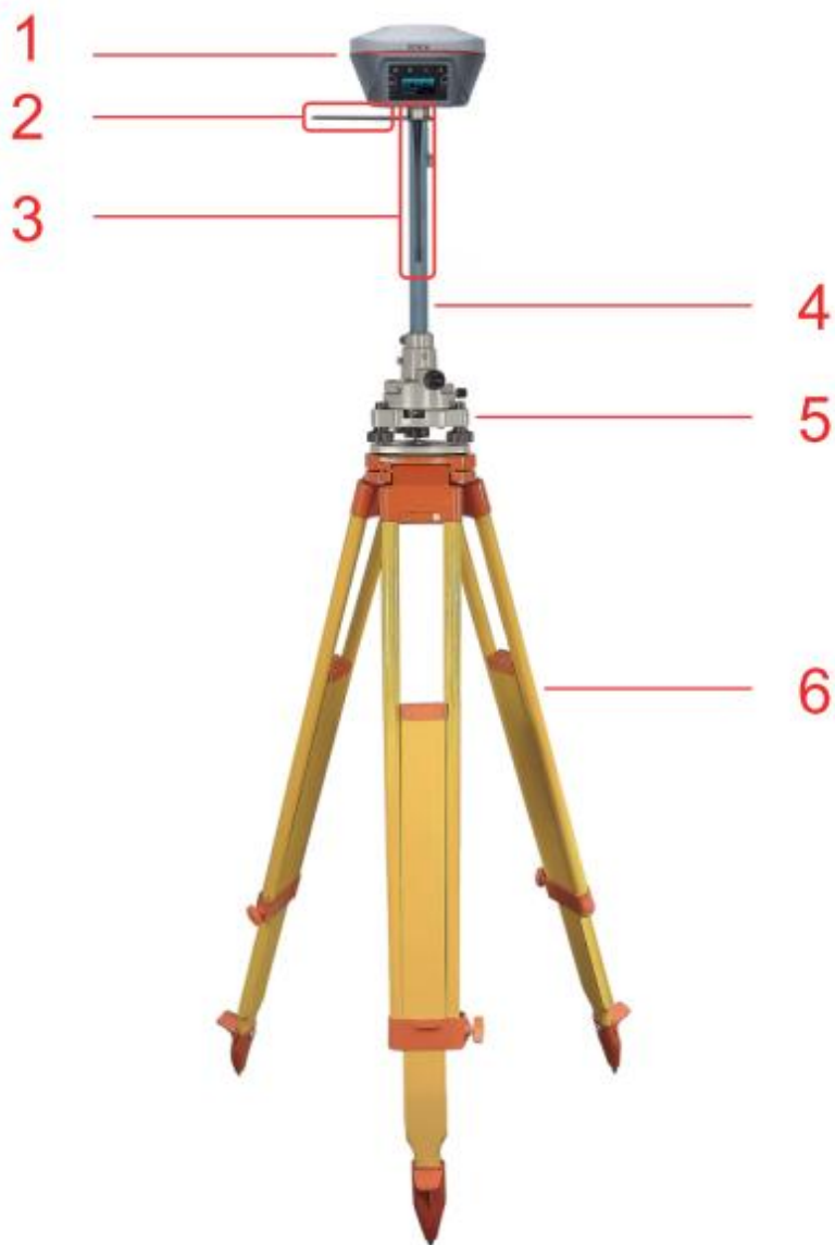
图 4.2 奥斯卡-TAP 作基准站-内置电台
