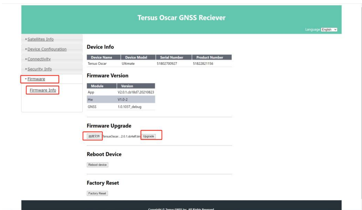
图 2.42 通过奥斯卡-TAPWIFI 网页进行升级
