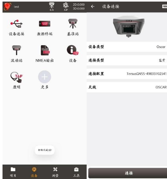
图 2.36 通过蓝牙连接奥斯卡-TAP
