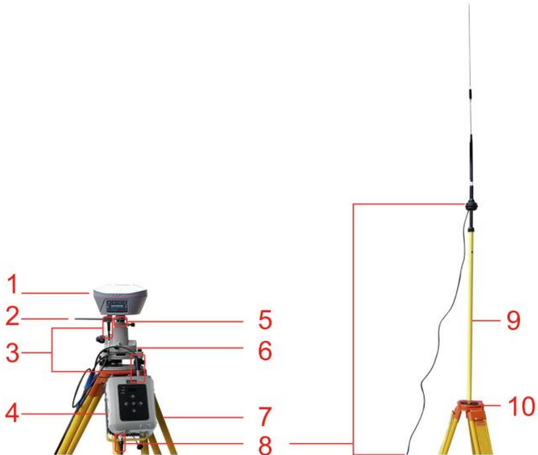
图 4.3 奥斯卡-TAP 作基准站-外置大电台
